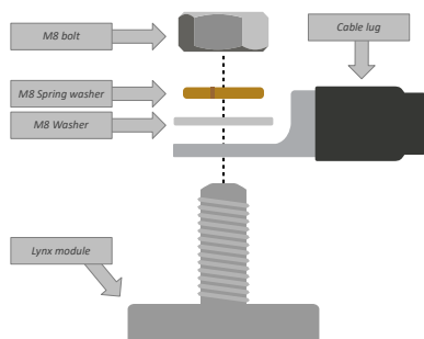
Figura 3. Secuencia de montaje correcta de los cables CC
