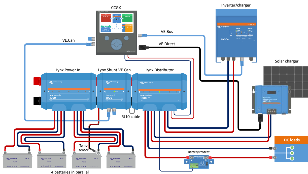
Sistema con Lynx Shunt VE.Can, baterías de plomo-ácido, un Lynx Shunt VE.Can y un Lynx Distributor
