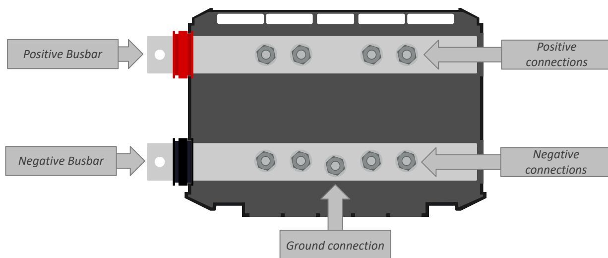
Elementos físicos internos del Lynx Power In
