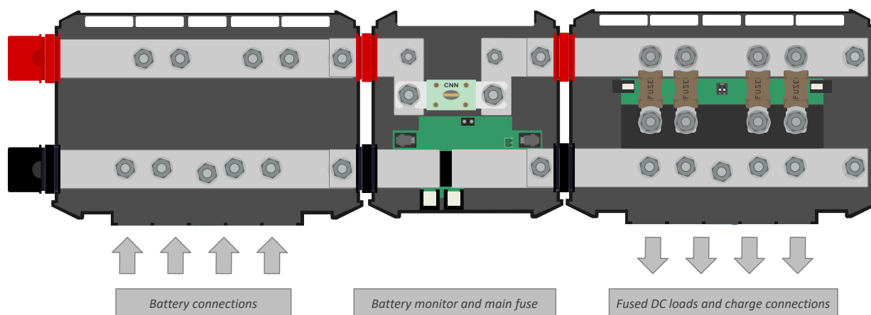
Módulos Lynx interconectados: Lynx Power In, Lynx Shunt VE.Can y distribuidor Lynx
